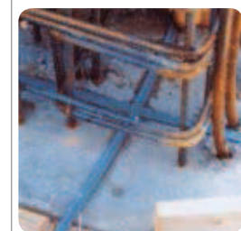
Eks. på tætning på Hydrotite® mellem pladsstøbt bundplade og væg.
